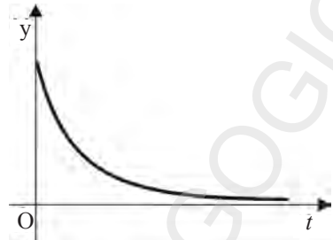
Fig. 1.24. Amortizare critică.
