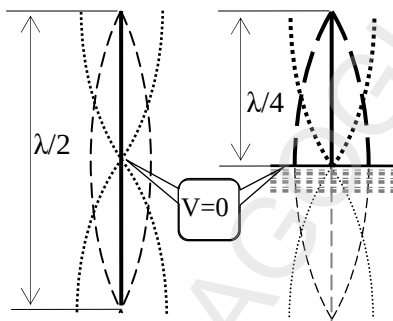
Fig. 3.59. Echivalența antenei sfert de undă cu cea semiundă
