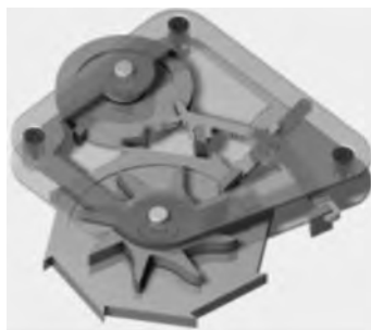
Fig. 1.30. Mecanismul ceasului
