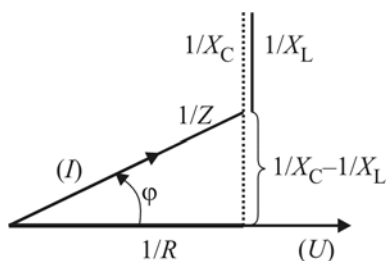
Fig. 3.36. a) Triunghiul susceptanțelor cu admitanța rezultantă, la circuitul paralel
