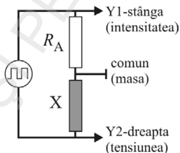
Fig. 3.4. Vizualizarea tensiunii și a intensității în procesele tranzitorii
