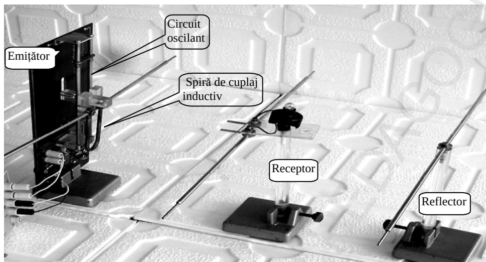
Fig. 3.62. Dispozitiv pentru emisia și recepția undelor electromagnetice. Se pot evidenția: modularea, reflexia, polarizarea și interferența undelor electromagnetice, precum și formarea undelor staționare.
