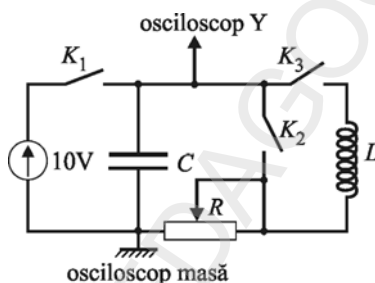
Fig 3.46. Vizualizarea pe osciloscop a descărcării condensatorului prin rezistor ( K_2 ) sau prin bobină ( K_3 )
