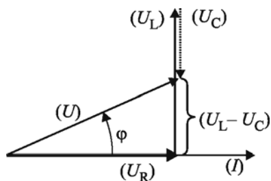
Fig. 3.21. Fazorii tensiunilor în circuitul serie, compuși după regula poligonului
