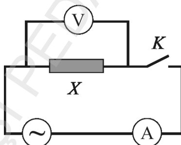
Fig. 3.3. Verificarea legii lui Ohm în curent alternativ.
