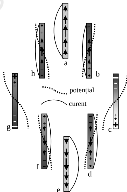
Fig. 3.56. Distribuția curentului și a potențialului în antenă
