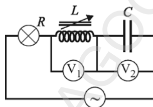
Fig. 3.28. Studiul rezonanței la circuitul serie
