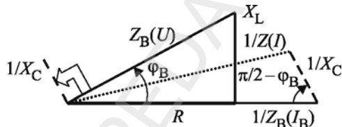
Fig. 3.44. Diagrama impedanței Z_B și a admitanțelor pentru fig. 3.41, 3.42
