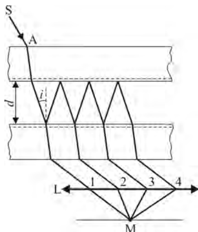
Fig. 4.32. Interferometrul Fabry-Perot
