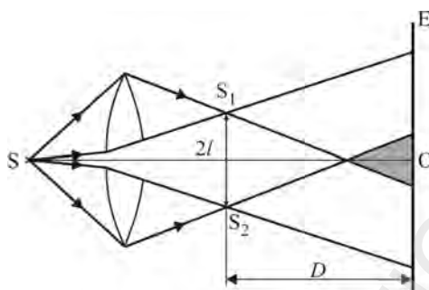
Fig. 4.23. Bilentilele Billet
