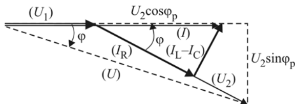
Fig. 3.39. Diagrama pentru obținerea lui U prin compunerea tensiunilor U_1 și U_2
