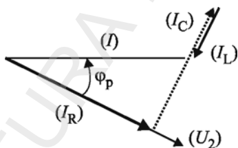
Fig. 3.38. Diagrama intensităților circuitului paralel, rotită cu -\varphi_p .
