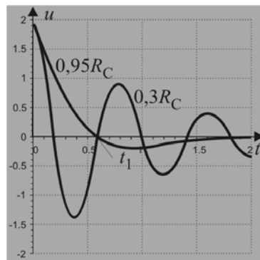
Fig. 3.52. Oscilații amortizate
