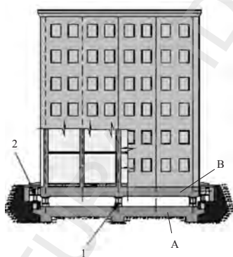
Fig. 1.32. Dispozitive de amortizare a undelor seismice: 1) verticale; 2) orizontale
