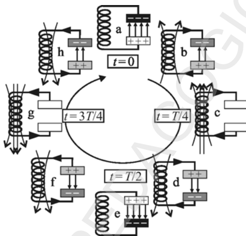
Fig. 3.49. Desfășurarea unei oscilații electromagnetice
