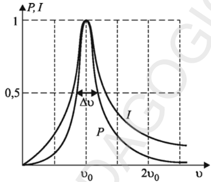
Fig. 3.30. Dependenta intensității și a puterii active de frecvență.
