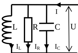
Fig. 3.34. Circuit RLC paralel cu bobină ideală
