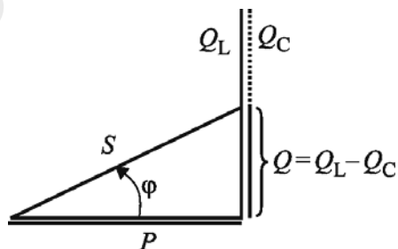
Fig. 3.27. Triunghiul puterilor pentru un circuit (serie) cu caracter inductiv
