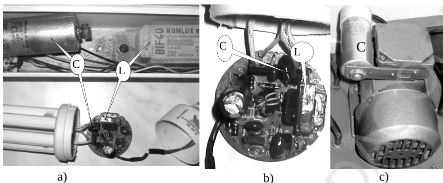
Fig. 3.33. a) Partea de alimentare a unei lămpi fluoerescente clasice (sus) comparată cu o lampă economică de aceeași putere (jos) L- balast, C- condensator pentru mărirea factorului de putere, b) convertizorul pentru alimentarea lămpii economice (detaliu), c) motor monofazat cu condensator
