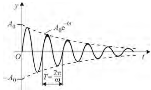
Fig. 1.25 – Mișcarea amortizată periodică
