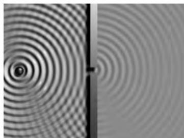
Fig. 2.7. Un punct de pe o suprafață de undă propagă unde identice cu cele produse de sursa primară
