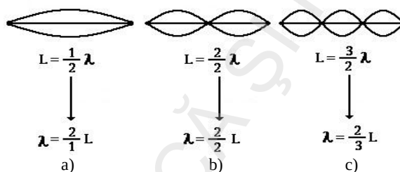
Fig. 2.31. Primele 3 moduri proprii de vibrație ale unei corzi de chitară
