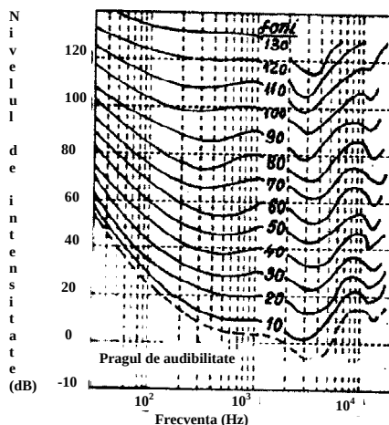
Fig. 2.28. Curbe de egal nivel de tărie
