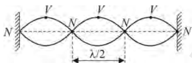
Fig. 2.21. Undă staționară într-un fir fixat la capete. V = ventru, N = nod
