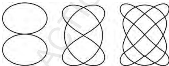
Fig. 1.21. Figuri Lissajous
