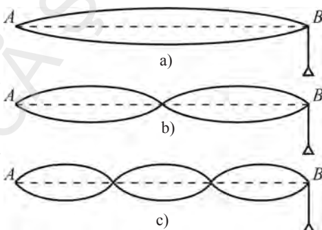
Fig. 2.25. Aspectul firului din figura 2.20 pentru prima, a doua și a treia armonică (a, b, c)
