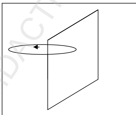
Fig. 5.6. „Secțiune Poincaré” în cazul unei mișcări periodice
