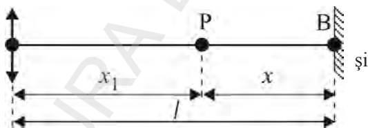
Fig. 2.22. În punctul P de pe fir se întâlnesc undele incidentă și reflectată
