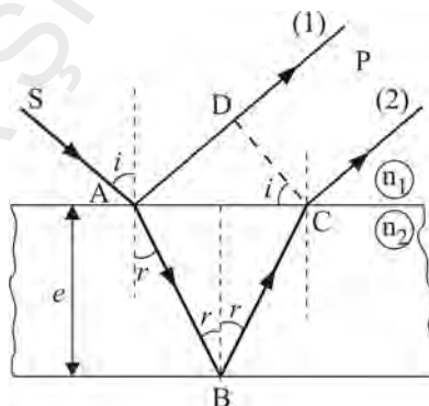
Fig. 4.25. Unde coerente obținute prin divizarea unei incidente. Lama cu fețe plan paralele
