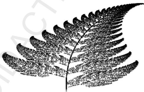
Fig. 5.15. Feriga lui Barnsley
