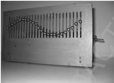
Fig. 2.3. Model de undă transversală
