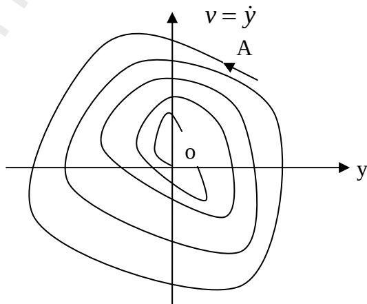
Fig. 5.3. Portretul din planul fazelor în cazul vibrației libere amortizate.
