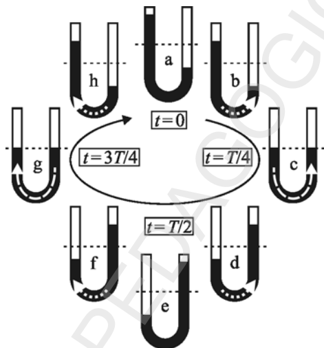
Fig. 3.51. Oscilațiile armonice ale unei coloane de lichid
