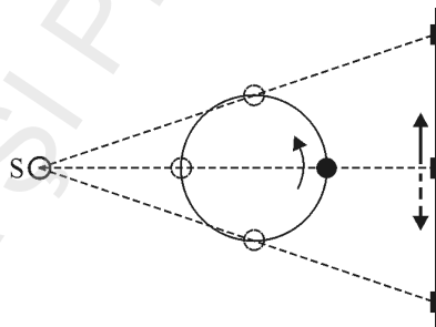
Fig. 1.2. Proiecția pe un ecran a unei mișcări circulare uniforme.
