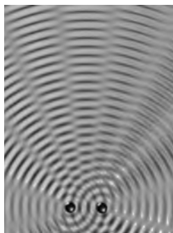
Fig. 2.17. Interferența undelor coerente dă o imagine de interferență stabilă
