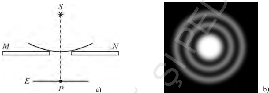
Fig. 4.34. a) Difrakția printr-un orificiu circular; b) frângele difrakției în cazul deschiderii circulare
