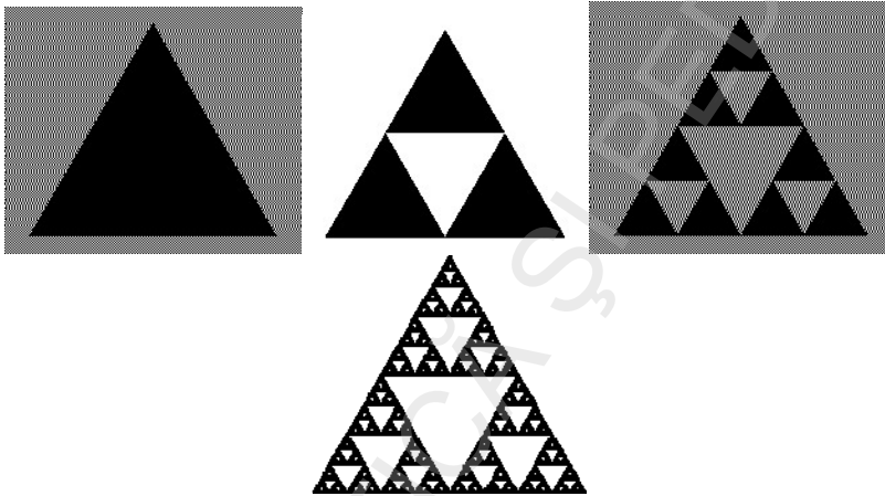
Fig. 5.11. Sita lui Sierpinsky
