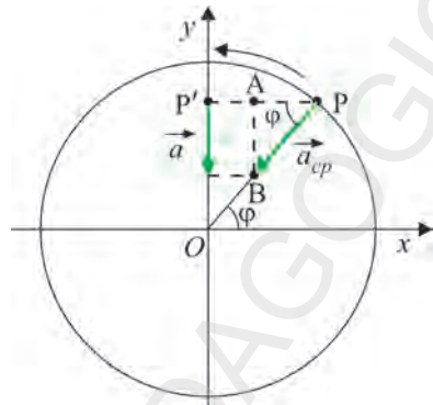
Fig. 1.6. Accelerația oscilatorului liniar armonic.
