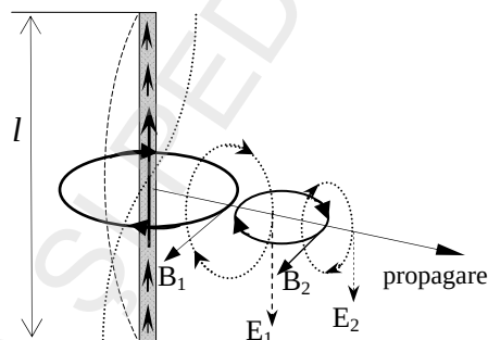
Fig. 3.57. Propagarea unei perturbații electrice prin intermediul câmpului electromagnetic
