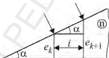
Fig. 4.27. Schemă pentru calculul interfranței
