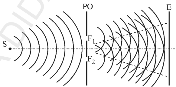
Fig. 4.15. Dispozitivul lui Young. Alcătuire
