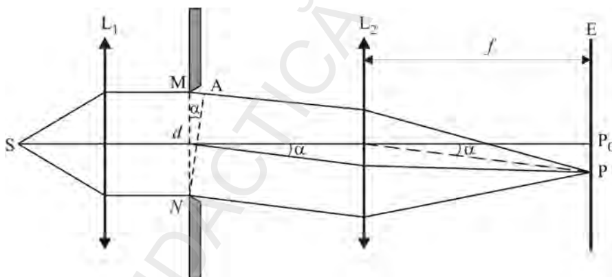
Fig. 4.37. Difrakția în lumină paralelă pe o fantă dreptunghiulară
