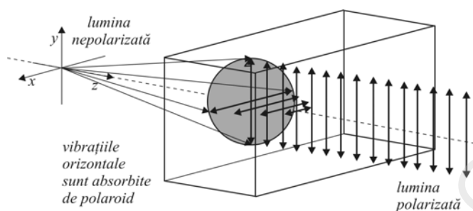
Fig. 4.50. Polarizarea prin absorbție selectivă
