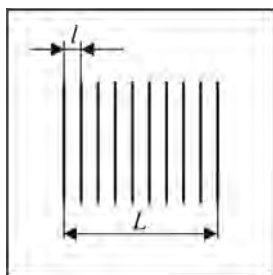
Fig. 4.39. Rețeaua de difracție
