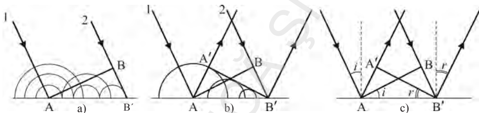
Fig. 2.9. Reflexia undelor
