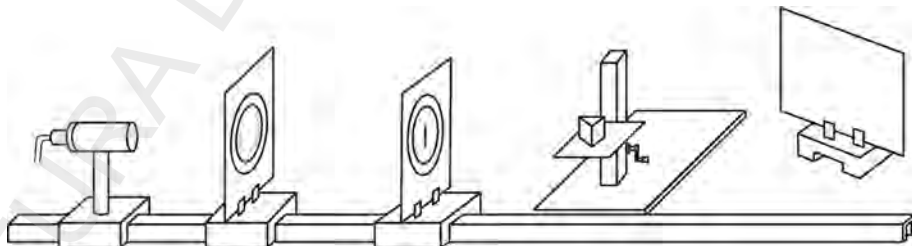
Fig. 4.9. Montaj pentru evidențierea dispersiei luminii
