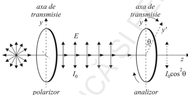
Fig. 4.53. Intensitatea fascicului emergent depinde de unghiul făcut de direcția de oscilație a vectorului luminos incident cu axa de transmisie a analizorului
