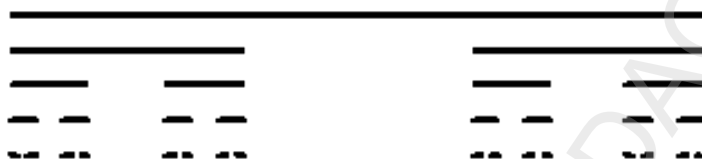
Fig. 5.9. Mulțimea lui Cantor
