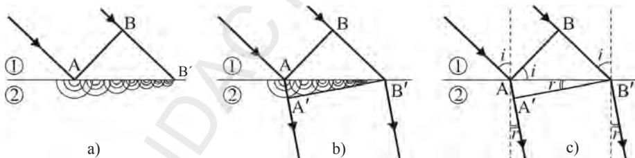
Fig. 2.11. Refracția undelor
