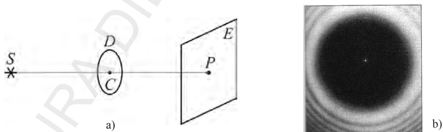
Fig. 4.35. a) Difrakția pe un disc circular opac; S – sursă; D – disc opac cu centrul în C ; E – ecran; P – punct pe axa SC ; b) – frânge de difrakție pentru un disc circular. În centrul imaginii este lumină
