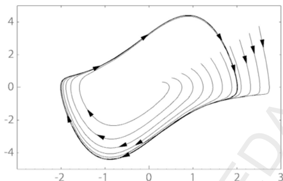
Fig. 5.4. Portretul din planul fazelor în cazul unui ciclu limită
