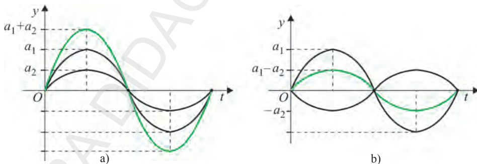
Fig. 1.17. Oscilația rezultantă: a) A = a_1 + a_2 ; b) A = |a_1 - a_2|
