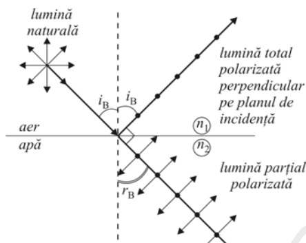
Fig. 4.47. Polarizarea total\ prin reflexie la inciden\ brewsterian\
