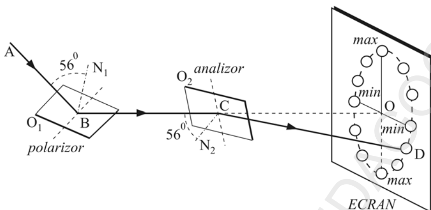
Fig. 4.54. Experimentul lui Malus. Rotirea analizorului duce la modificarea intensității luminoase a fasciculului transmis
