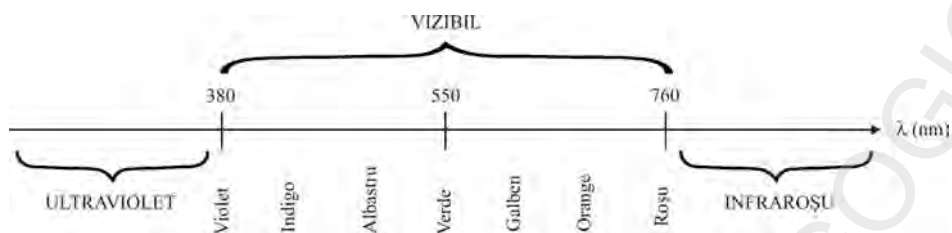
Fig. 4.1. Spectrul radiațiilor optice
