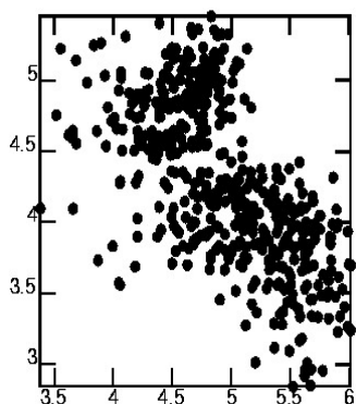
Fig. 5.8. „Secțiunea Poincaré” în cazul unei mișcări haotice
