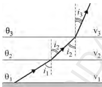
Fig. 2.12. La amiază, vara \theta_1 > \theta_2 > \theta_3 și v_1 > v_2 > v_3 . Atunci i_1 > i_2 > i_3 și raza sonoră deviază în sus
