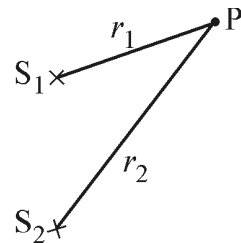
Fig. 4.14. Două surse de lumină punctiforme S_1 și S_2 care emit radiații paralele de aceeași frecvență
