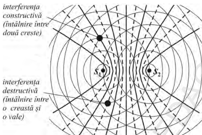
Fig. 2.16. Franje de interferență. Liniile pline arată locurile unde creste provenite de la sursa S_1 întâlnesc creste de la S_2 , cu obținerea de creste duble (interferență constructivă)
