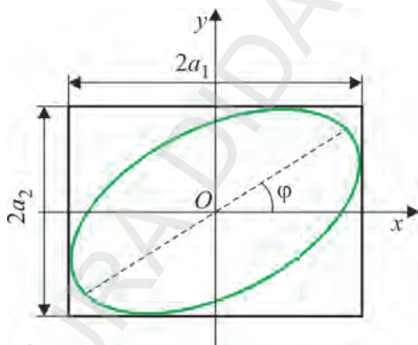
Fig. 1.20. Traiectoria unui mobil supus simultan acțiunii a două oscilații perpendiculare de aceeași frecvență
