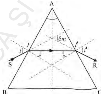
Fig. 4.6. În cazul deviației minime, traiectul luminos S I I' R este simetric în raport cu planul bisector al unghiului A al prisme
