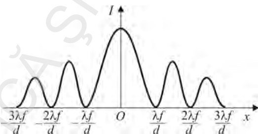
Fig. 4.38. Distribuția intensității luminoase în funcție de distanță la difracția pe o fantă
