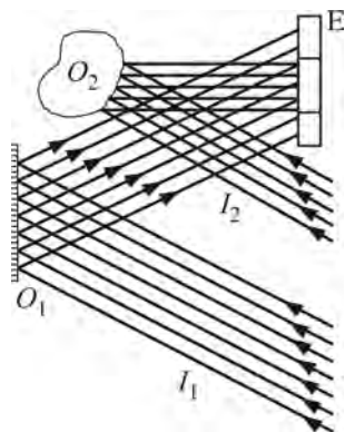
Fig. 4.44. Principiul obținerii hologramei
