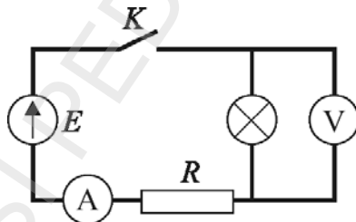
Fig. 3.1. Studiul regimului tranzitoriu pentru bec
