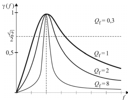
Fig. 3.31. Caracteristici de frecvență pentru diverse valori ale factorului de calitate (nivelul \frac{\sqrt{2}}{2} evidențiază lărgimea de bandă)
