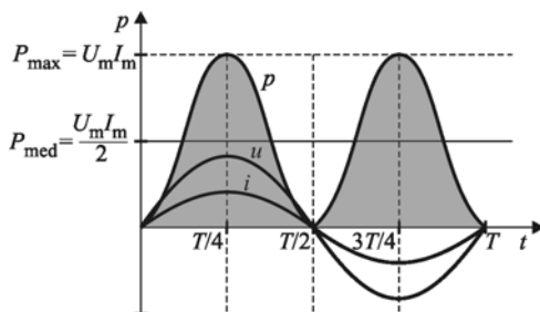
Fig. 3.15. Puterea instantanee pe rezistor în decursul unei perioade
