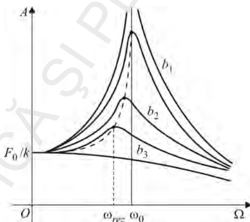
Fig. 1.26. Curbe de rezonanță ( b_1 < b_2 < b_3 ).
