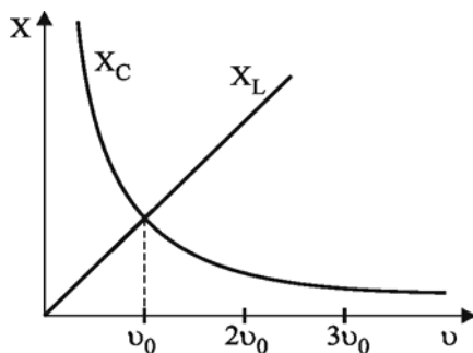
Fig. 3.14. Dependența reactanțelor de frecvență ( \nu_0 – frecvența de rezonanță)
