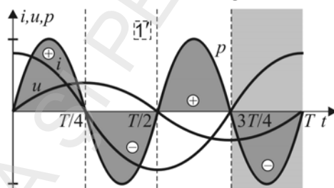
Fig. 3.17. Puterea instantanee pentru condensator
