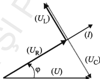
Fig. 3.24. Diagrama fazorială a unui circuit serie având caracter capacitiv, în care (U) este fazor de referință
