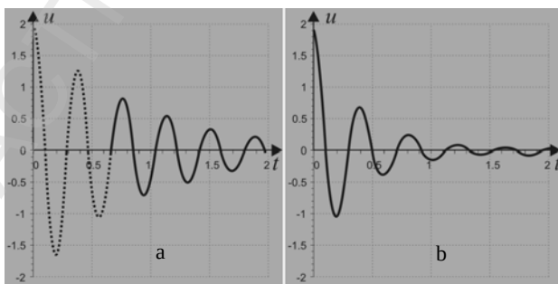
Fig. 3.48. Descărcarea condensatorului pe o bobină a) slab amortizată; b) puternic amortizată
