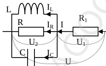
Fig. 3.37. Circuit RLC paralel, legat în serie cu un rezistor
