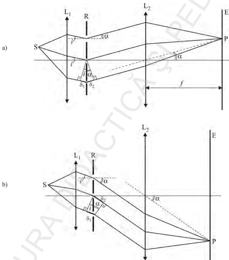
Fig. 4.40. Obținerea experimentală a difracției pe rețea
