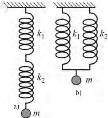
Fig. 1.9. Resorturi serie sau paralel
