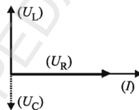
Fig. 3.19. Fazorii tensiunilor din circuitul serie puși în aceeași origine
