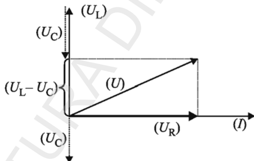
Fig. 3.20. Compunerea fazorilor după regula paralelogramului pentru circuitul serie
