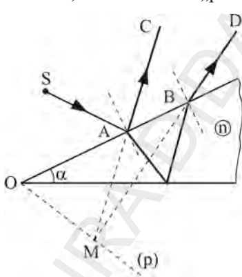
Fig. 4.26. Pana optică
