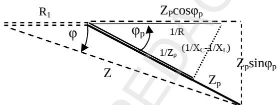
Fig. 3.40. Diagrama impedanțelor R_1 și Z_p , pentru obținerea lui Z
