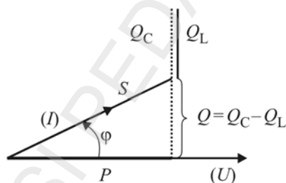
b) Triunghiul puterilor pentru circuitul paralel
