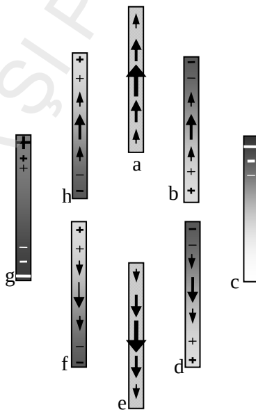
Fig. 3.55. Desfășurarea oscilației libere în antenă
