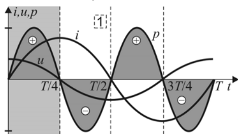
Fig. 3.16. Puterea instantanee pentru bobină. Comparați 1 cu 1' din 3.17
