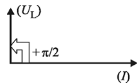
Fig. 3.12. Fazorii tensiunii și intensității pentru bobină (intensitatea este referință)
