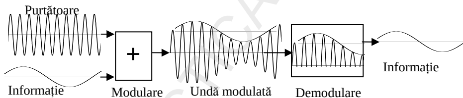
Fig. 3.61. Transmiterea informației cu ajutorul undelor modulate în amplitudine
