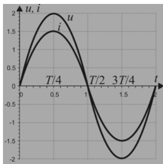
Fig. 3.8. La rezistor tensiunea și intensitatea sunt în fază
