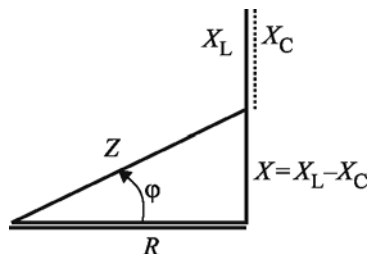
Fig. 3.22. Triunghiul impedanței unui circuit serie cu caracter inductiv
