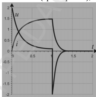
Fig. 3.6. Regimul tranzitoriu pentru bobina reală
