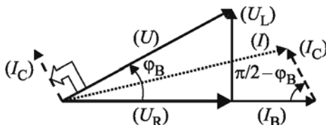
Fig. 3.43. Diagrama fazorială a bobinei reale ( U_R, U_L, U, I_B ), la care s-a atașat, în raport cu U , diagrama condensatorului ( I_C, U )
