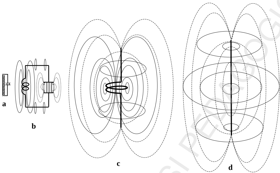
Fig. 3.53 Trecerea de la circuitul oscilant închis (a) la antena (d). Punctat sunt reprezentate liniile electrice, continuu- cele magnetice. (Dacă desenul (a) este la scara 1:1, atunci (d) trebuie considerat la scara 1:100)
