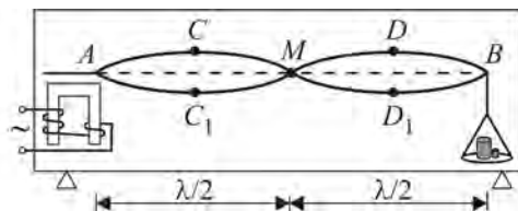
Fig. 2.20. Dispozitiv pentru producerea undelor staționare
