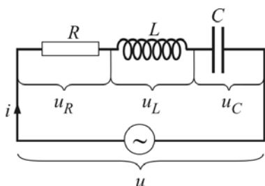
Fig. 3.18. Circuitul RLC serie
