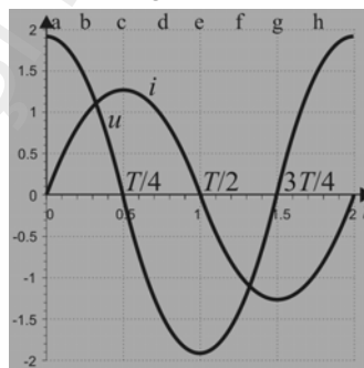
Fig. 3.50. Oscilațiile tensiunii și intensității sunt defazate cu \pi/2
