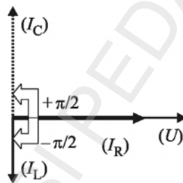
Fig. 3.35. Fazorii intensităților din circuitul paralel puși în aceeași origine
