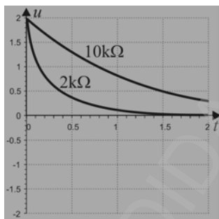
Fig. 3.47. Descărcarea aperiodică a condensatorului
