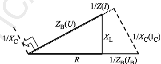
Fig. 3.45. Diagrama circuitului LC real la rezonanță: (I) și (U) sunt suprapuse
