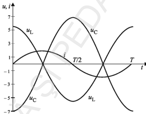
Fig. 3.25. Graficele tensiunilor u_L și u_C în cazul unui circuit serie (se observă că, între ele, acestea sunt în opoziție de fază și defazate cu \pm \pi/2 față de i )
