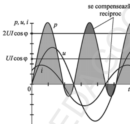
Fig. 3.26. Puterea instantanee în funcție de timp (i defazat cu \pi/4 în fața lui u)
