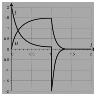
Fig. 3.7. Încărcarea și descărcarea condensatorului (regim tranzitoriu)
