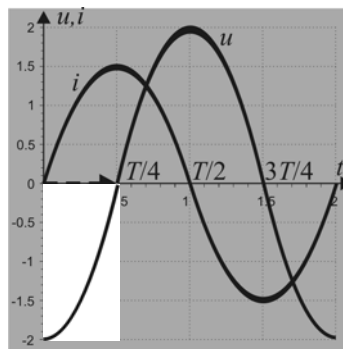
Fig. 3.10. La condensator curentul este în fața tensiunii: dacă deplasăm graficul i spre dreapta cu T/4 (îl întârziem), u și i vor fi în fază.
