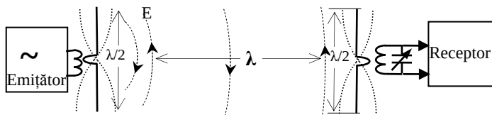
Fig. 3.60. Emiterea și receptarea undelor electromagnetice
