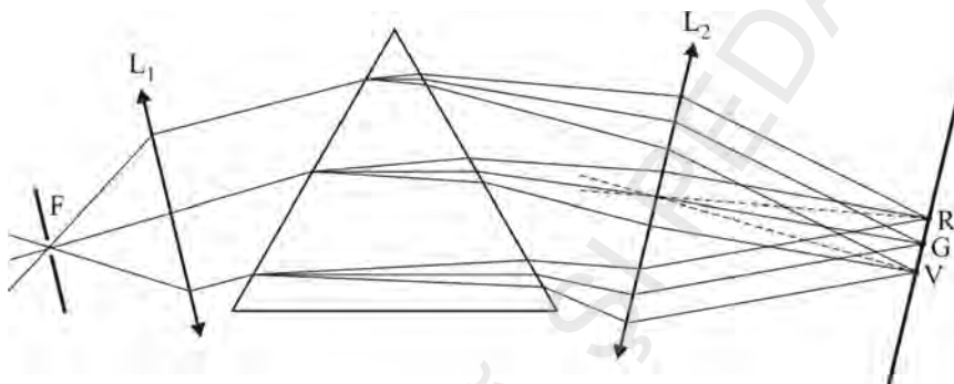
Fig. 4.13. Schema unui aparat spectral cu prismă
