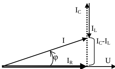
Fig. 3.36. Diagrama intensităților pentru un circuit paralel
