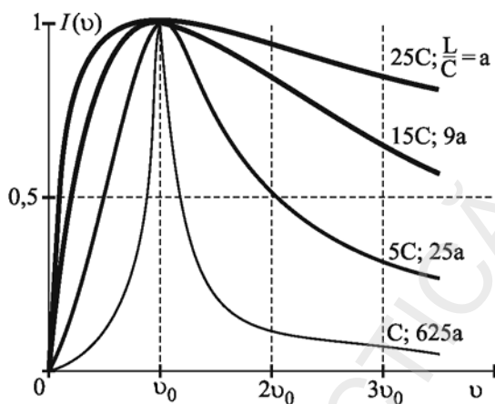
Fig. 3.29. Curbe de rezonanță pentru aceeași rezistență și aceeași frecvență de rezonanță, dar pentru capacități și inductanțe diferite
