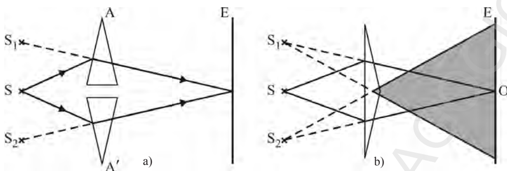
Fig. 4.22. Biprismă Fresnel
