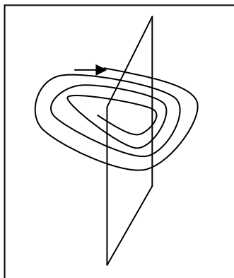
Fig. 5.7. „Secțiune Poincaré” în cazul unei mișcări oscilatorii amortizate
