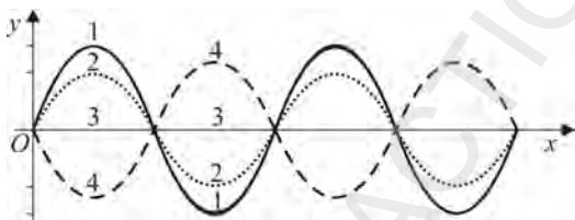
Fig. 2.24. Coarda la momente diferite
