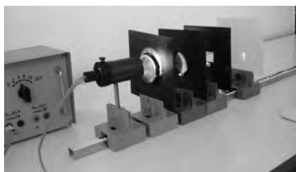
Fig. 4.41. Montaj experimental pentru studiul rețelei de difracție
