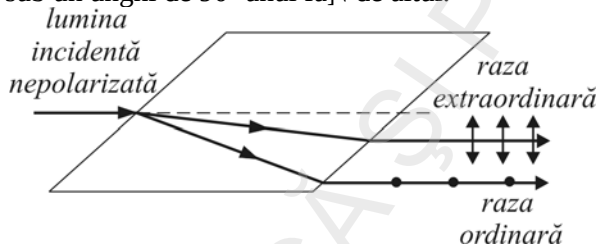
Fig. 4.48. Dubla refrac \backslash ie a luminii n cristalul de spat de Islanda. Cele dou \backslash raze (ordinar \backslash și extraordinar \backslash ) sunt liniar polarizate, dar direc \backslash iile de oscila \backslash ie ale vectorilor lumino \backslash i sunt reciproc perpendiculare
