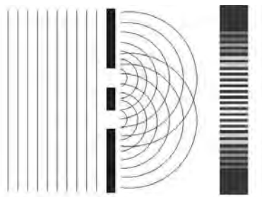
Fig. 4.20. Obținerea franjelor paralele și echidistante
