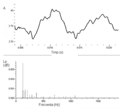
Fig. 2.29 b. Sunet muzical
