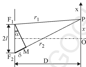
Fig. 4.16. Între două raze care interferează există o diferență de drum \delta
