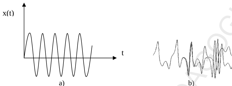
Fig. 5.1. Vibrograme. a) mișcare periodică; b) mișcare haotică.
