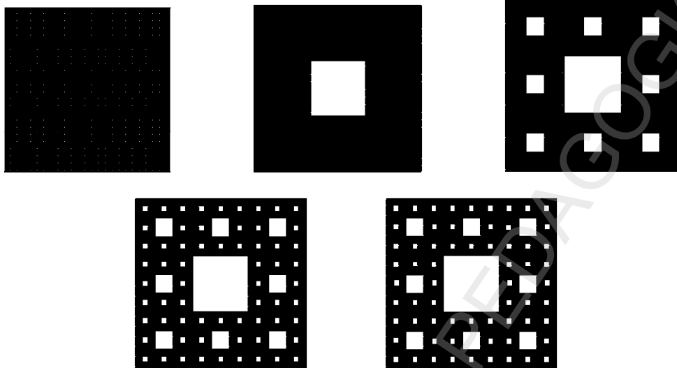
Fig. 5.13. Covorul lui Sierpinsky
