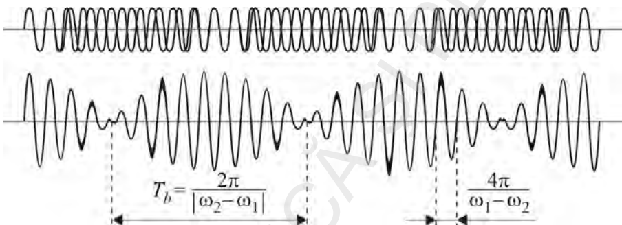
Fig. 1.18. Fenomenul bătilor
