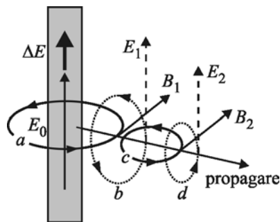
Fig. 3.54. Producerea și propagarea câmpului electromagnetic
