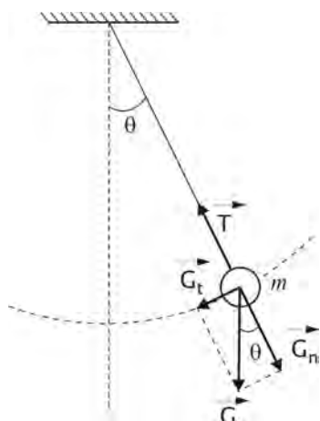
Fig. 1.12. Forțele care acționează asupra pendulului
