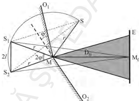
Fig. 4.21. Oglinzile lui Fresnel
