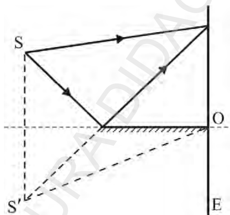
Fig. 4.24. Oglinda lui Lloyd
