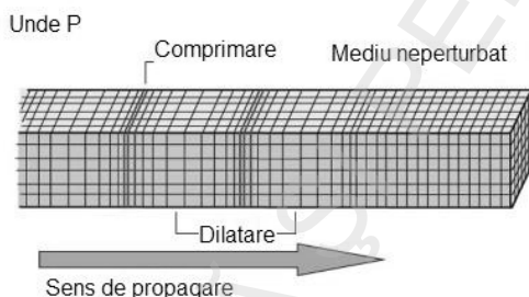
Fig. 2.39. Unde P
