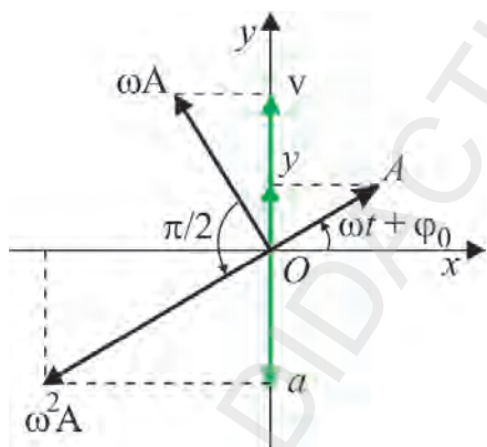
Fig. 1.15. Reprezentarea fazorială a elongației, vitezei și accelerației oscilatorului liniar armonic
