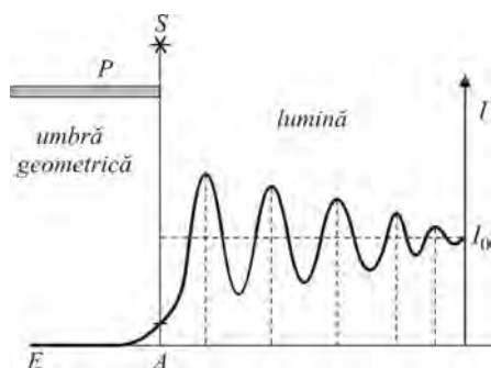
Fig. 4.36. Difrakția la marginea unui paravan
