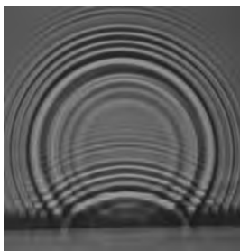
Fig. 2.8. Reflexia undelor
