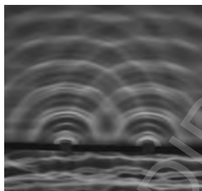
Fig. 2.14. Interferența a două unde
