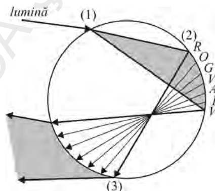
Fig. 4.12. Dispersia luminii într-o picătură de apă.
