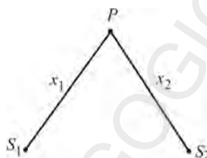
Fig. 2.15. Perturbațiile produse de sursele S_1 și S_2 ajung într-un punct arbitrar P după ce au parcurs distanțele x_1 respectiv x_2
