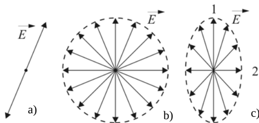
Fig. 4.46. a) lumină total polarizată; b) lumină naturală; c) lumină parțial polarizată
