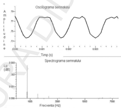
Fig. 2.29 a. Sunet pur
