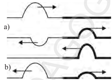
Fig. 2.10. Reflexia unei perturbații transversale
