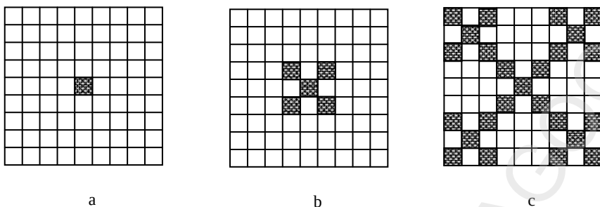
Fig. 5.17. Modelul lattice Witten-Sander
