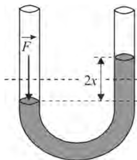
Fig. 1.10. Coloana oscilantă de lichid
