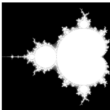
Fig. 5.16. Mulțimea Mandelbrot
