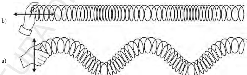
Fig. 2.4. Propagarea unei unde: a) transversal; b) longitudinal într-un resort elastic
