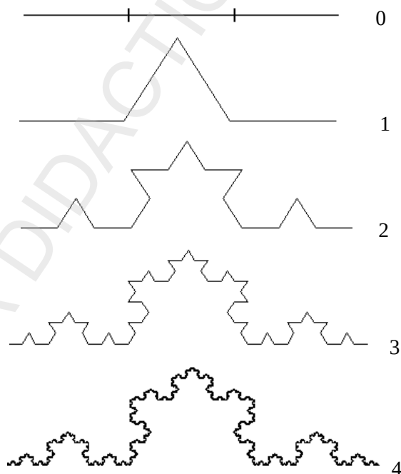
Fig. 5.10. Curba lui von Koch
