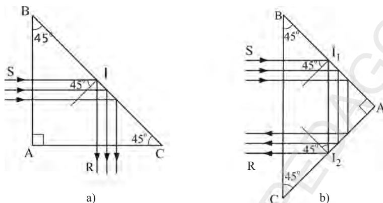
Fig. 4.7. Prisme cu reflexie totală.
