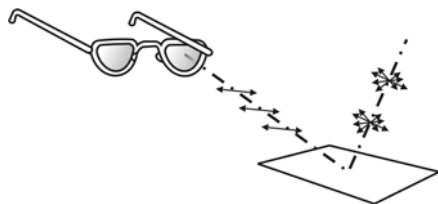
Fig. 4.55. Filtrul polarizant al ochelariilor elimină strălucirea neplăcută a luminii reflectate sub anumite unghiuri
