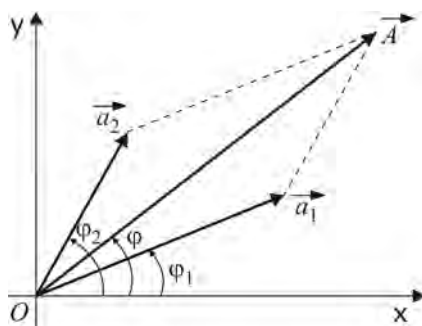
Fig. 1.16. Compunerea oscilațiilor prin metoda fazorială
