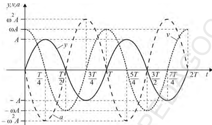
Fig. 1.14. Graficele elongației, vitezei și accelerației oscilatorului liniar armonic ( \varphi_0=0 )
