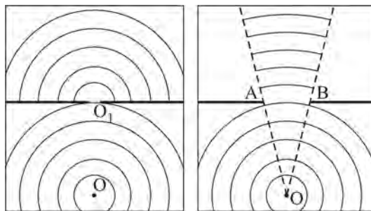
Fig. 2.13. a) d \approx \lambda ; b) d \gg \lambda
