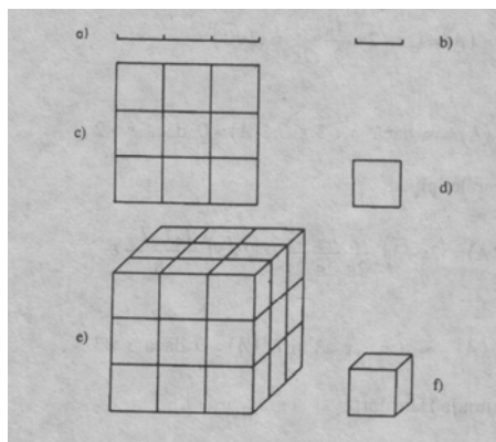
Fig. 5.12. Dimensiunea de autosimilaritate
