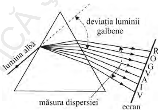
Fig. 4.8. Dispersia produsă de o prismă. Ansamblul culorilor de pe ecran se numește spectru.
