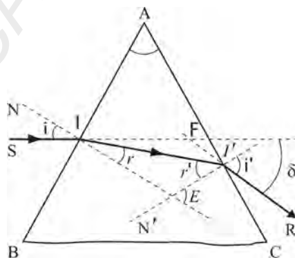
Fig. 4.5. Mersul unei raze de lumină într-o secțiune principală a unei prisme.
