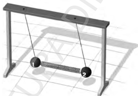
Fig. 1.28. Pendule simple cuplate.
