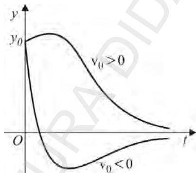
Fig. 1.23. Mișcare amortizată aperiodică.
