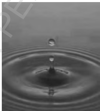
Fig. 2.1. Formarea undelor pe suprafața apei
