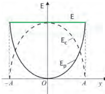
Fig. 1.11. Energia oscilatorului armonic
