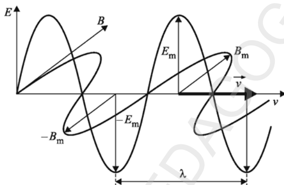
Fig. 3.58. Vectorii E și B ai unde plane la un moment dat
