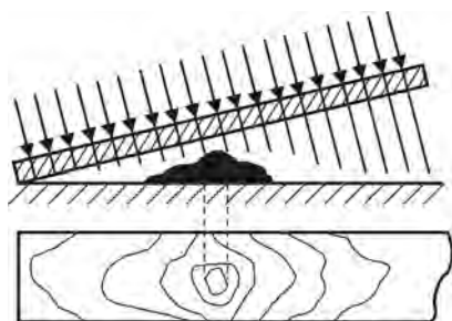
Fig. 4.28. Deformarea franjelor de egală grosime datorită abaterilor de la planeitate
