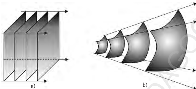
Fig. 2.5. a) undă plană; b) undă sferică
