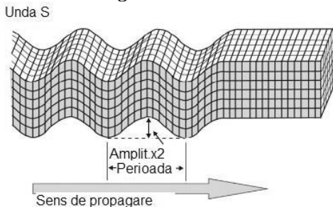
Fig. 2.40. Unde S
