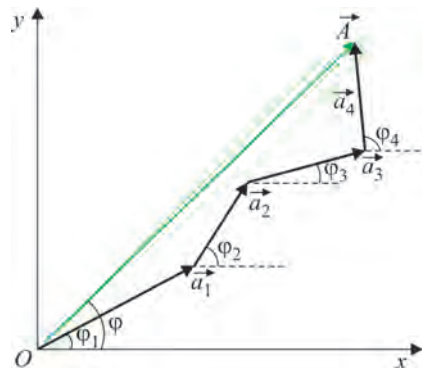
Fig. 1.19. Compunerea fazorială a mai multor vibrații paralele de aceeași frecvență
