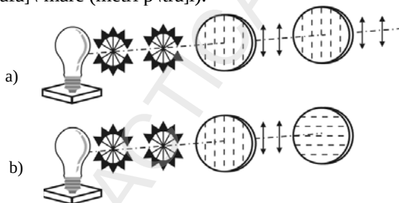
Fig. 4.51. Folosirea polaroizilor. a) Când axele de transmisie sunt paralele, lumina trece (fiind polarizată liniar); b) când axele sunt perpendiculare, obținem extincția luminii
