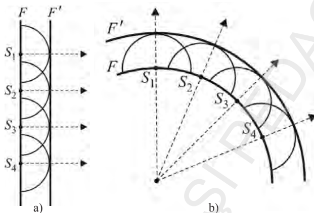
Fig. 2.6. Construirea fronturilor de undă pentru unde plane (a) și unde sferice (b)
