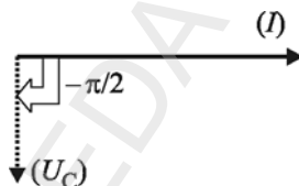
Fig. 3.13. Fazorii tensiunii și intensității pentru condensator (I – fazor de referință)
