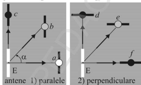
Fig. 3.63. Amplitudinea semnalului emis depinde de direcția ( \alpha ) de emisie (a,b,c) și de orientarea relativă a antenelor (d,e,f) (polarizarea este orizontală)
