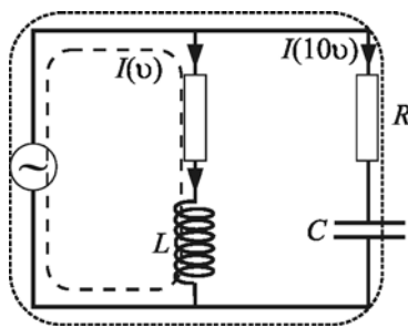
Fig. 3.32. Separarea componentelor de joasă (prin bobină) și înaltă frecvență (prin condensator)
